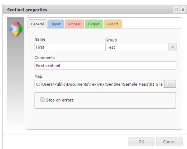
Abbildung: Plug-In-Einstellungen
