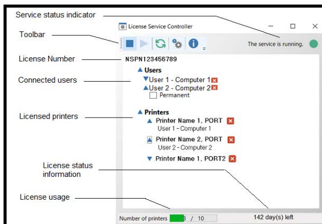
Figure 4 bis : Contrôleur de service de licence pour les licences limitées par imprimantes
