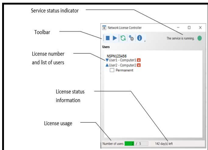
Abbildung 4: Service Control-Hauptfenster
