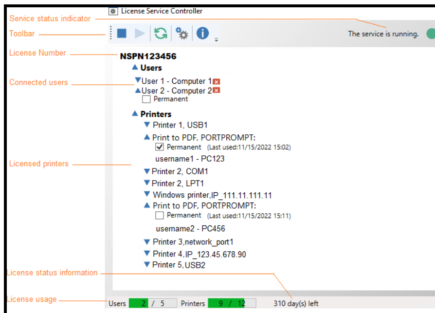
Figura 4: Finestra principale di License Service Controller
